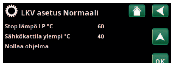
Valikko "Edistyneempi/Asetukset/Aset. Ylätankki/LKV-ohjelma/LKV-ohjelma Normaali".
