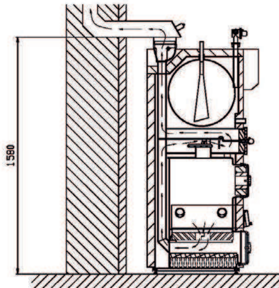
MÄTTSKISS RÖKRÖRSMONTAGE
