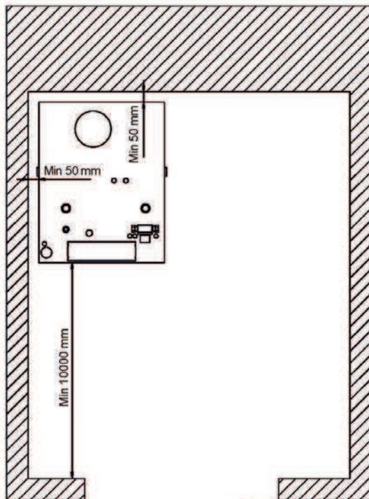
MÄTTSKISS PANNANS UPPSTÄLLNING
