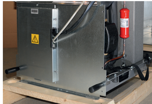
6. Asenna kylmämoduuli takaisin kahvojen ja nostoremmin avulla, irrota kahvat ja remmi, kiinnitä ruuvit, sähköpistokkeet ja letkut.
