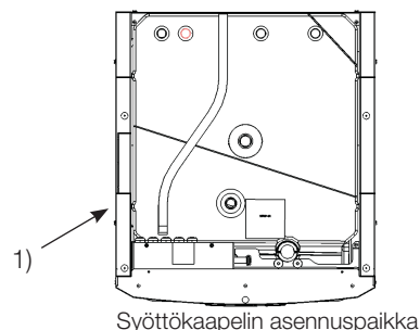
Syöttökaapelin asennuspaikka
