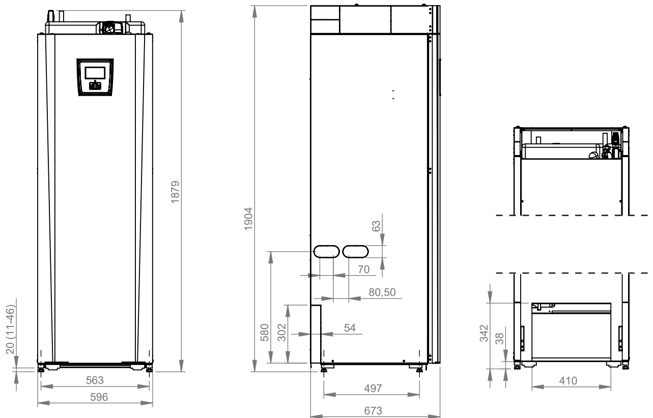
Høj model - CTC EcoZenit i255H
