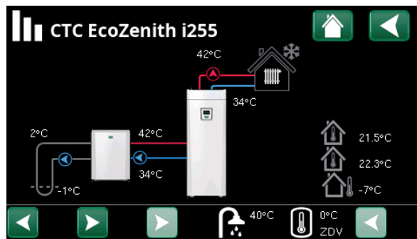
Na zaslonu so prikazane informacije o delovanju s priključeno toplotno črpalko CTC EcoPart.
