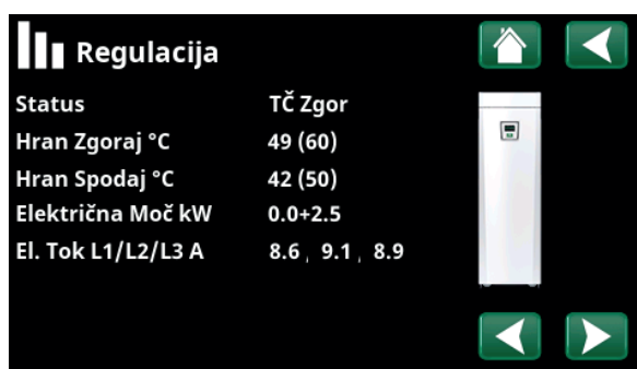
Meni: »Podatki o delovanju, krmilna enota«. Kliknite puščice ali podsajte za preklop med krmilno enoto in toplotno črpalko.
