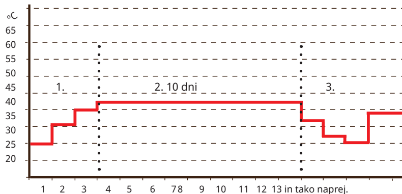
Primer za Način 2 z nastavljenno vrednostjo »Sušenje Estriha Temp °C«: 37.
