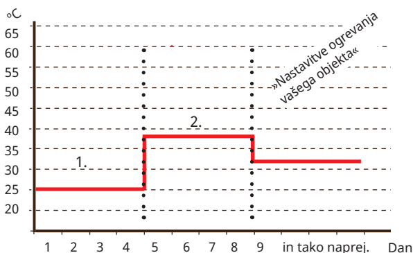
Primer za Način 1 z nastavljenno vrednostjo »Sušenje Estriha Temp °C«: 38.
