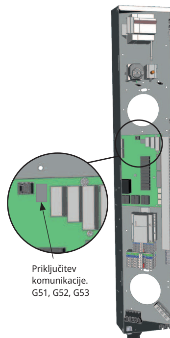
Priključna omarica EcoZenith
