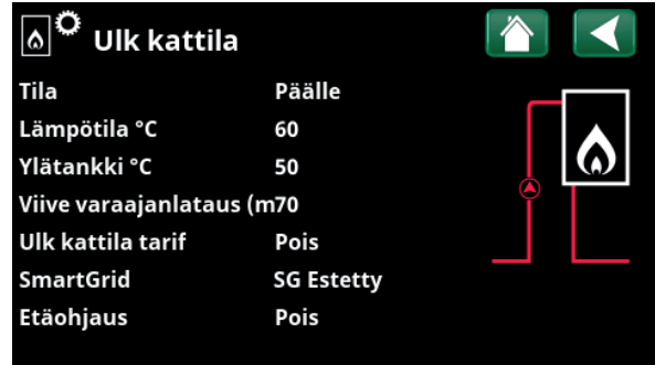
Valikko "Käyttötiedot/Ulk. kattila".
