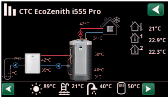
Päävalikkosivu "Käyttötiedot" neste-/vesilämpöpumppu CTC EcoPart kytkettynä. Kun pumput ovat käynnissä, myös kuvan pumppusymbolit kiertyvät.
