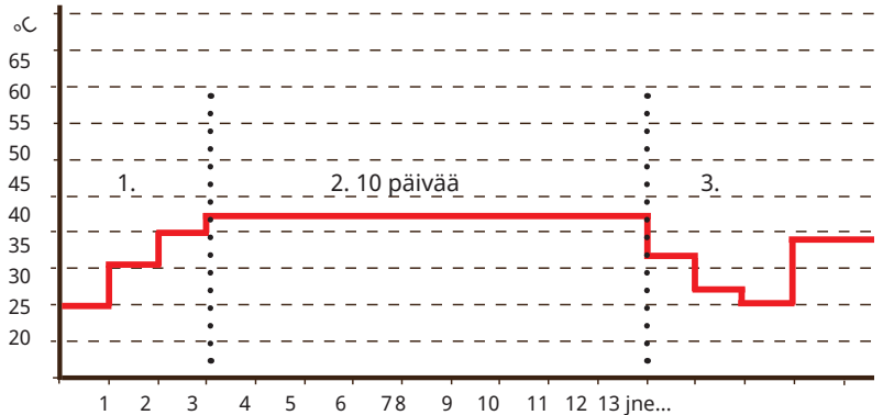
Esimerkki tilalle 2, jossa asetettu arvo toiminnolle "Lattiatomiminto lämp. °C": 37.
