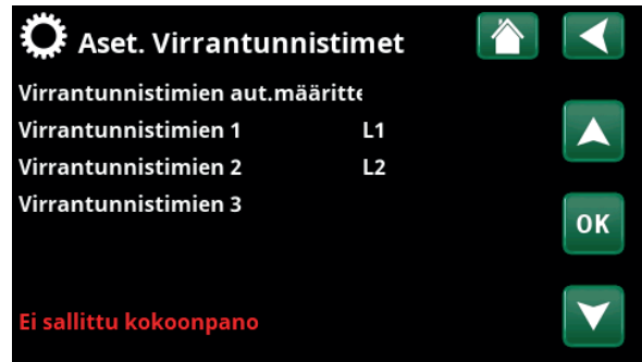
Valikko "Edistyneempi/Asetukset/Virrantunnistimet".
