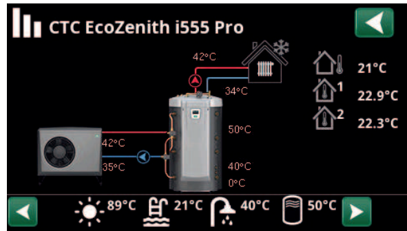
Päävalikkosivu "Käyttötiedot" ilma-/vesilämpöpumppu CTC EcoAir kytkettynä. Kun pumput ovat käynnissä, myös kuvan pumppusymbolit kiertyvät.
